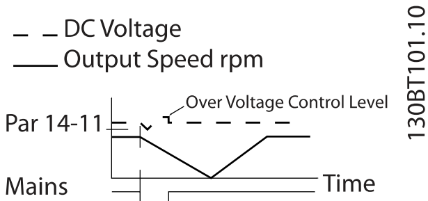
图 3.2: 受控减速—主电源短时间故障。 减速直到停止, 接着加速到参考值。
