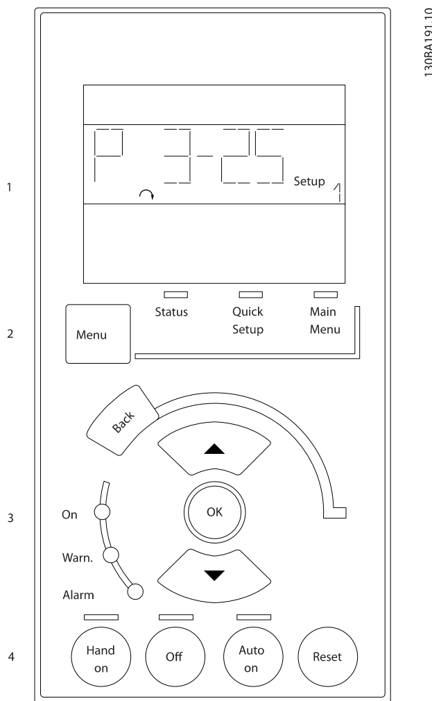
图 2.1: 数字式 LCP (NLCP)
