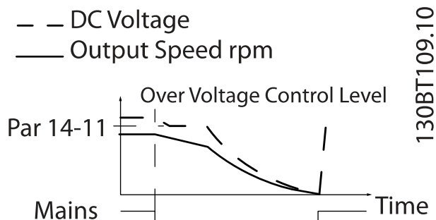
图 3.5: 借能运行, 主电源长时间故障。 一旦系统中的能量过低, 电动机就会惯性停车。
