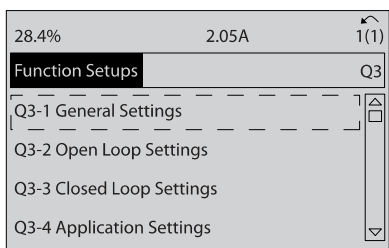
图 2.9: 步骤 4: 功能设置选项随即显示。选择 Q3-1 一般设置。按 [OK] (确定)。
