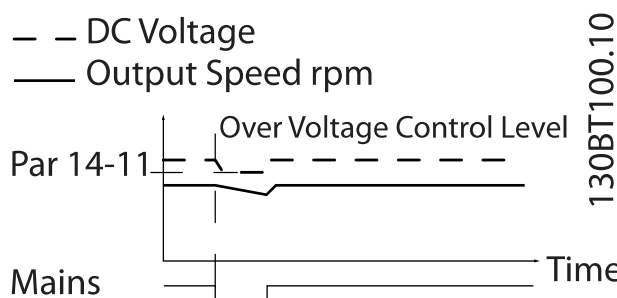
图 3.4: 借能运行, 主电源短时间故障。 只要系统中的能量允许, 便保持运行。
