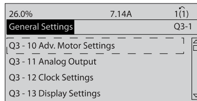
图 2.10: 步骤 5: 使用向上/向下导航键向下滚动到目标选项, 比如 Q3-11 模拟输出。按 [OK] (确定)。
