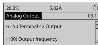
图 2.11: 步骤 6: 选择参数 6-50。按 [OK] (确定)。
