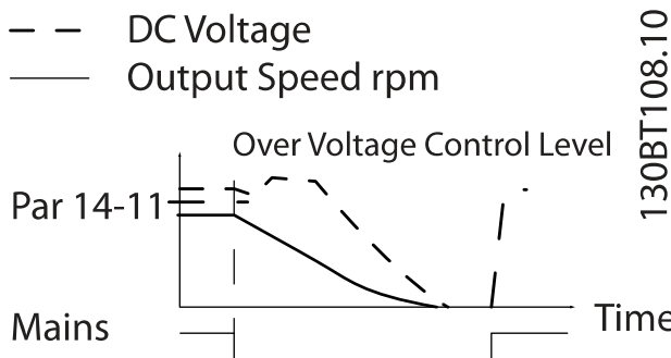
图 3.3: 受控减速, 主电源长时间故障。 只要系统中的能量允许, 便进行减速, 之后电动机将惯性停车。
