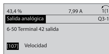
Ilustración 2.12 Paso 7: use las teclas de navegación arriba / abajo para seleccionar entre las distintas opciones. Pulse [OK] (Aceptar).
