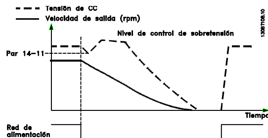
Ilustración 3.3 Deceleración controlada, fallo más largo de alimentación. Deceleración tan larga como lo permita la energía almacenada en el sistema, y luego motor a inercia.
