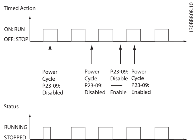
Ilustración 3.6 Diagrama de prueba de reactivación
