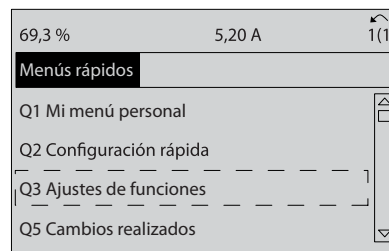
Ilustración 2.8 Paso 3: use las teclas de navegación arriba / abajo para desplazarse por las configuraciones de funciones. Pulse [OK] (Aceptar).
