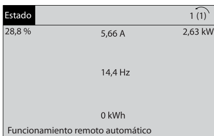
Ilustración 2.6 Paso 1: encienda el convertidor de frecuencia (el LED amarillo se ilumina).
