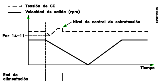
Ilustración 3.2 Deceleración controlada - fallo breve alimentación. Deceleración hasta parar seguida por aceleración hasta referencia.
