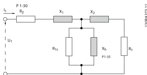
Ilustración 3.1 Diagrama equivalente del motor para un motor asíncrono
