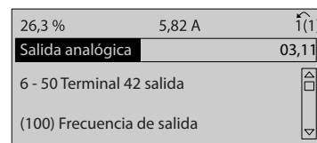
Ilustración 2.11 Paso 6: seleccione el par. 6-50. Pulse [OK] (Aceptar).
