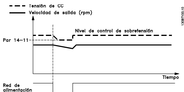
Ilustración 3.4 Energía regenerativa, fallo breve de aliment. Mantener tanto como lo permita la energía almacenada en el sistema.
