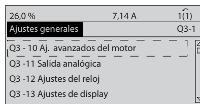
Ilustración 2.10 Paso 5: use las teclas de navegación arriba / abajo para desplazarse hasta, p. ej., Q3-11 Salidas analógicas . Pulse [OK] (Aceptar).
