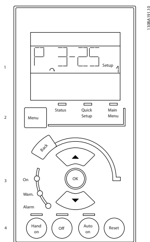
Ilustración 2.1 Panel numérico LCP (NLCP)
