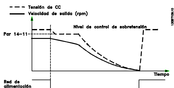
Ilustración 3.5 Energía regenerativa, fallo más largo de aliment. El motor queda en inercia tan pronto como se detecte que la energía del sistema es demasiado baja.
