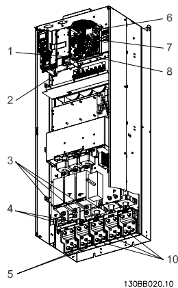
Bild 4.8: Compact IP 00 (chassi) med frånskiljare, säkring och RFI-filter, ramstorlek E2
