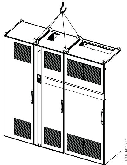
Bild 3.6: Rekommenderad lyftmetod, enhetsstorlek F3.
