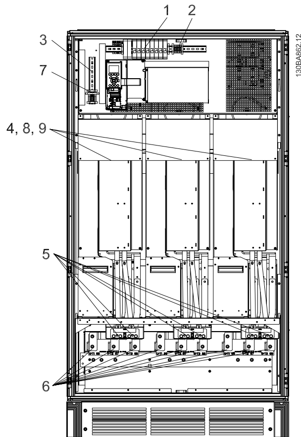
Bild 4.12: Växelryktarskåp, ramstorlek F2 och F4
