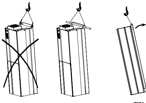
Afbeelding 3.24: Hijsmethode voor wandbevestiging van omvormer
