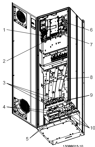
Afbeelding 4.1: Compact IP 21 (NEMA 1) en IP 54 (NEMA 12), framegrootte D1
