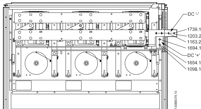
Afbeelding 3.26: Klemposities – Regen-klemmen – F2 en F4
