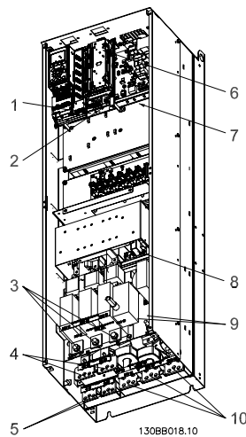
Afbeelding 4.4: Compact IP 00 (Chassis) met werkschakelaar, zekering en RFI-filter, framegrootte D4
