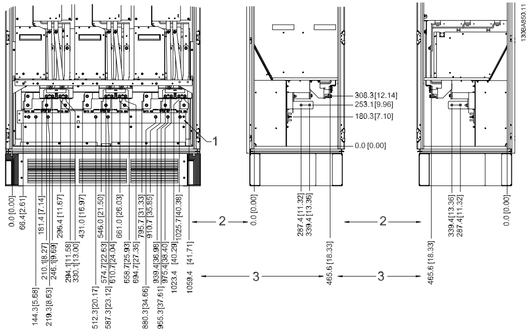
Afbeelding 3.25: Klemposities – inverterkast – F2 en F4 (vooraanzicht, zijanzicht links en rechts). De doorvoerplaat bevindt zich op 42 mm onder niveau '0.0'.
