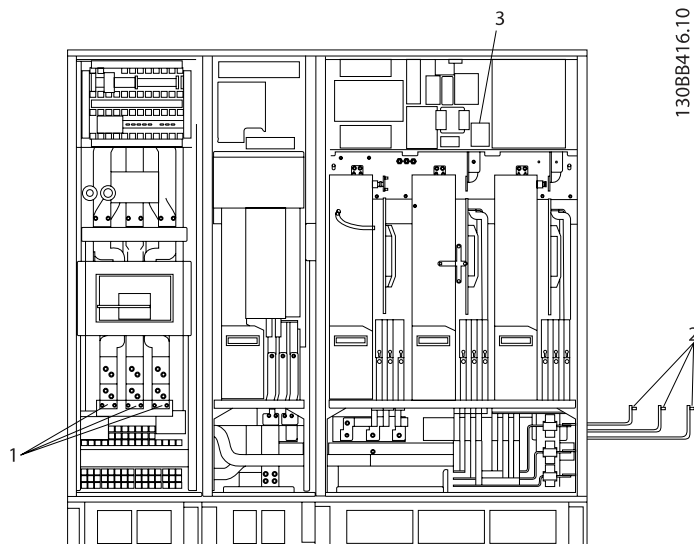
图 4.30: 有源滤波器, 机架规格 F17
