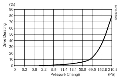
图 4.22: E 机架的降容与 压力变化 (大风扇) P355-P450 变频器气流: 850 cfm (1445 m 3 /h)
