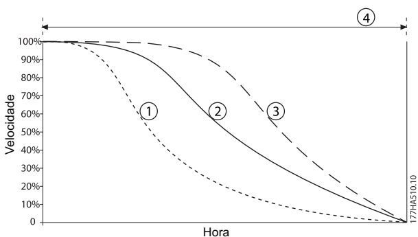
1. Desaceleração antecipada 2. Desaceleração constante 3. Desaceleração postergada 4. Tempo de parada (Par. 1-10)
