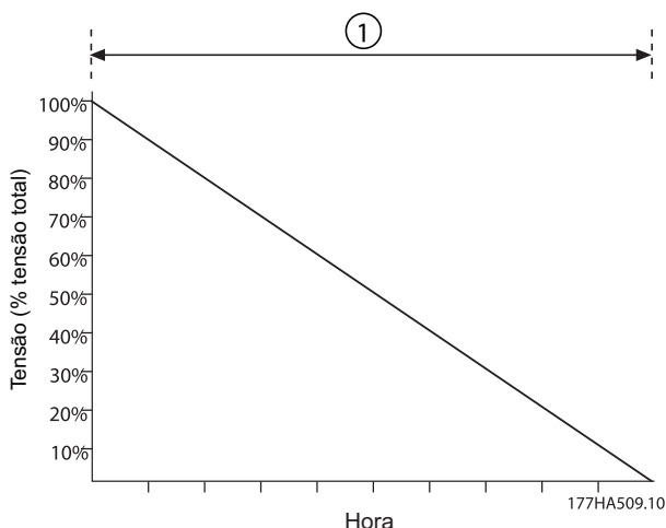
1: Tempo de parada (Par. 1-11)
