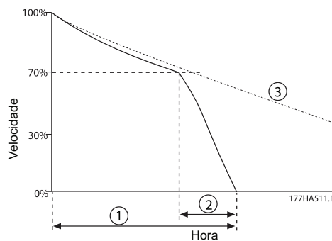
1: Tempo de parada (Par. 1-11) 2: Tempo de frenagem (Par. 1-16) 3: Tempo de parada por inércia
