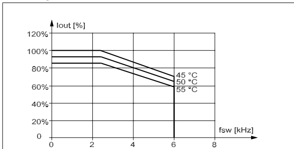
Εικόνα 10.11: Υποβιβασμός του I_{out} για διαφορετική τιμή T_{AMB, MAX} για το περίβλημα D σε 600 V, με χρήση 60 AVM σε τρόπο λειτουργίας κανονικής ροής (110% υπερ-ροπή). Σημείωση: Δεν ισχύει για P315.
