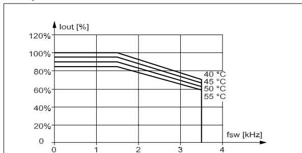
Εικόνα 10.14: Υποβιβασμός του I_{out} για διαφορετική τιμή T_{AMB, MAX} για το περίβλημα D σε 600 V, με χρήση SFAVM σε τρόπο λειτουργίας κανονικής ροής (110% υπερ-ροπή). Σημείωση: P315 μόνο .
