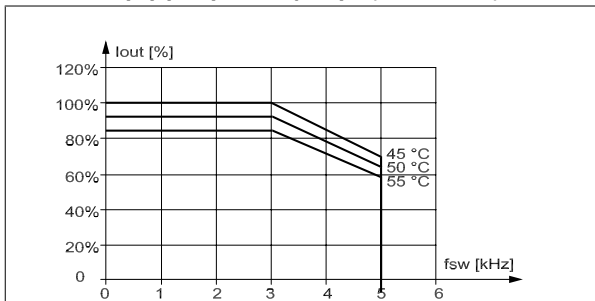
Εικόνα 10.13: Υποβιβασμός του I_{out} για διαφορετική τιμή T_{AMB, MAX} για το περίβλημα D σε 600 V, με χρήση 60 AVM σε τρόπο λειτουργίας κανονικής ροής (110% υπερ-ροπή). Σημείωση: P315 μόνο .
