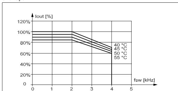
Εικόνα 10.16: Υποβιβασμός του I_{out} για διαφορετική τιμή T_{AMB, MAX} για περίβλημα E σε 480 V, με χρήση SFAVM σε τρόπο λειτουργίας κανονικής ροής (110% υπερ-ροπή)
