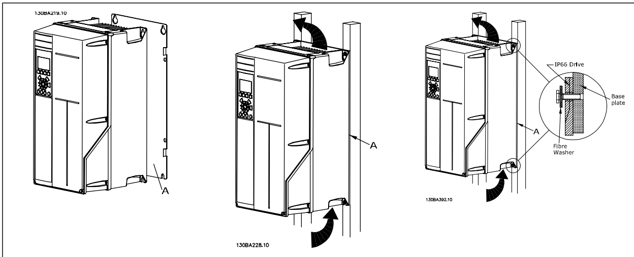
Πίνακας 4.2: Κατά την τοποθέτηση πλαισίου μεγέθους A5, B1, B2, B3, B4, C1, C2, C3 και C4 σε μη σταθερό πίσω τοίχο, μαζί με το ρυθμιστή στροφών πρέπει να παρέχεται και μια πίσω πλάκα A λόγω ανεπαρκούς κυκλοφορίας ψυχρού αέρα πάνω από την ψύκτρα.
