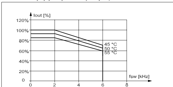
Εικόνα 10.15: Υποβιβασμός του I_{out} για διαφορετική τιμή T_{AMB, MAX} για το περίβλημα E σε 480 V, με χρήση 60 AVM σε τρόπο λειτουργίας κανονικής ροής (110% υπερ-ροπή)
