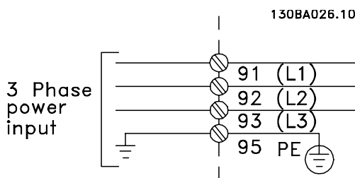
Εικόνα 5.5: Ακροδέκτες για δίκτυο ρεύματος και γείωση.
