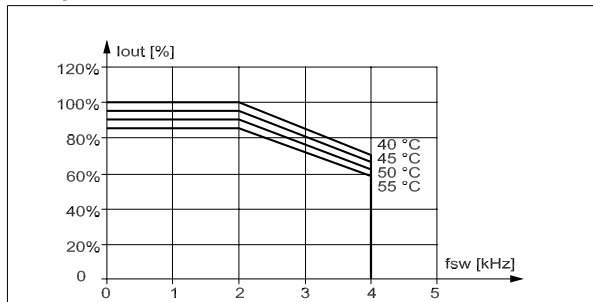
Εικόνα 10.12: Υποβιβασμός του I_{out} για διαφορετική τιμή T_{AMB, MAX} για το περίβλημα D σε 600 V, με χρήση SFAVM σε τρόπο λειτουργίας κανονικής ροής (110% υπερ-ροπή). Σημείωση: Δεν ισχύει για P315.
