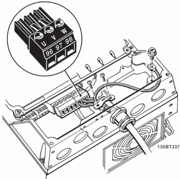
그림 5.22: 먼저 모터 접지를 차단한 다음, 모터 U, V 및 W 와이어를 단자에 놓고 조이십시오. EMC 클램프 아래로 모터 케이블의 외부 절연이 제거되었는지 확인하십시오.
