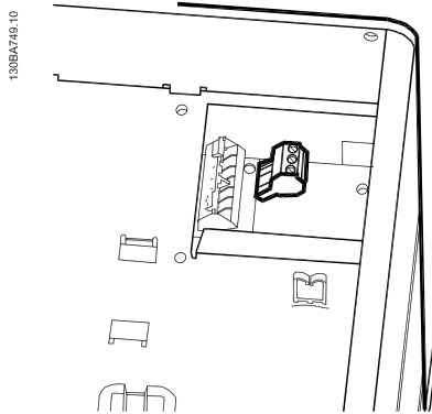
그림 5.40: C3 및 C4의 릴레이 연결용 단자. 주파수 변환기의 오른쪽 상단에 있습니다.
