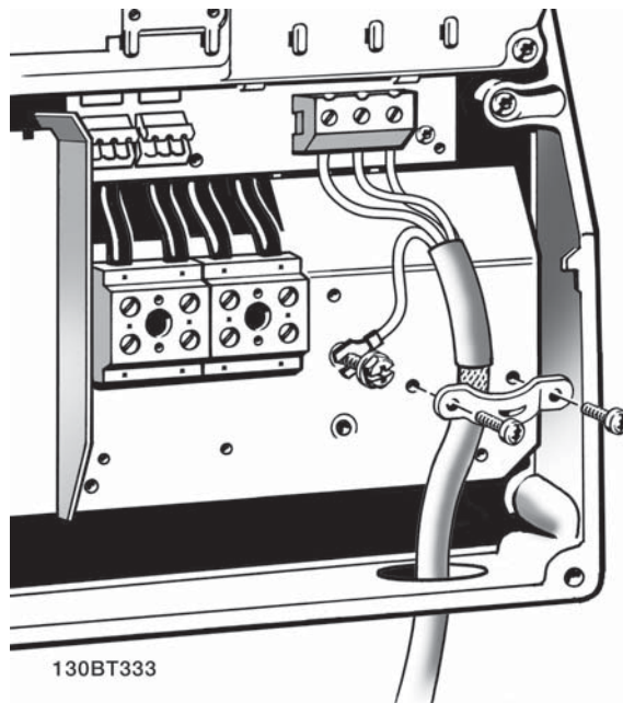
그림 5.23: 먼저 모터 접지를 차단한 다음, 모터 U, V 및 W 와이어를 단자에 놓고 조이십시오. EMC 클램프 아래로 모터 케이블의 외부 절연이 제거되었는지 확인하십시오.
