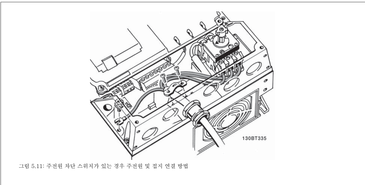
그림 5.10: 주전원 차단 스위치가 없는 경우 주전원 및 접지 연결 방법 케이블 클램프가 사용된다는 점에 유의하십시오.
