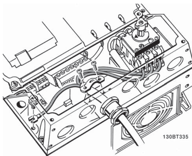
图 5.11: 如何使用主电源断路器连接主电源和接地。
