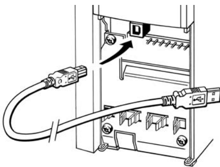
图 7.10: 有关控制电缆连接的信息，请参阅有关控制端子的章节。
