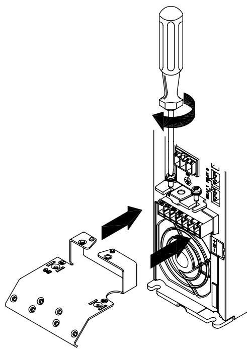
图 5.6: 首先, 将两个螺钉安装到固定板上, 然后将其滑动入位并完全拧紧。
