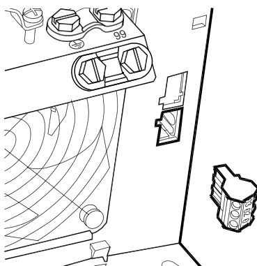
Afbeelding 5.34: Klemmen voor relaisaansluiting B3. In de fabriek is slechts één relaisingang aangebracht. Verwijder de uitbreekpoort als een tweede relais nodig is.
