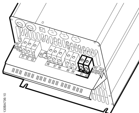
Afbeelding 5.31: Aansluitklem remweerstand/-kabel voor C3.
