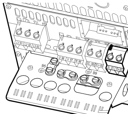
Afbeelding 5.30: Aansluitklem remweerstand/-kabel voor B4.
