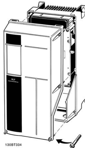
Afbeelding 5.38: Toegang tot de stuurklemmen voor behuizing A5, B1, B2, C1 en C2
