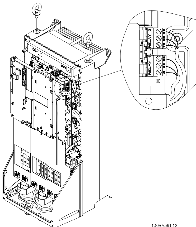
Afbeelding 5.33: Klemmen voor relaisaansluiting (behuizing C1 en C2).
