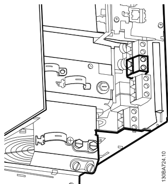
Afbeelding 5.29: Aansluitklem remweerstand/-kabel voor B3.
