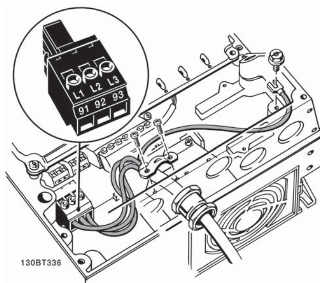
Afbeelding 5.6: Aansluiting op net en aarding zonder netschakelaar. Er is echter wel een kabelklem gebruikt.
