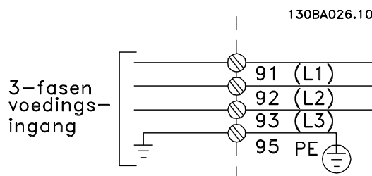
Afbeelding 5.1: Klemmen voor netvoeding en aarding.
