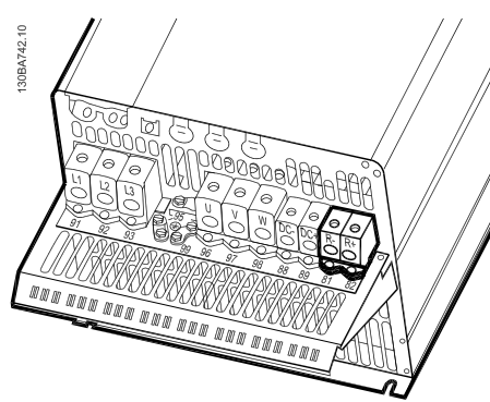
Afbeelding 5.32: Aansluitklem remweerstand/-kabel voor C4.
