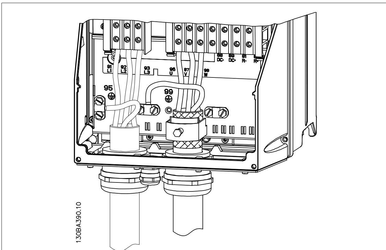
Ilustração 5.22: Primeiro, faça a terminação do terra do motor, em seguida, instale os fios U, V e W no terminal e aperte. Garanta que a isolamento externa do cabo do sob a braçadeira de EMC seja removida.
