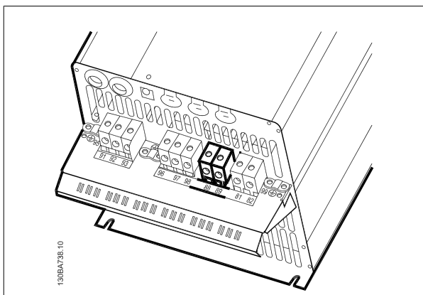
Ilustração 5.27: Conexões do barramento CC para o gabinete metálico C3.
