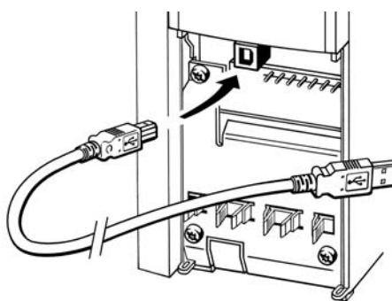
Ilustração 7.10: Para as conexões de cabo de controle, consulte a seção Terminais de Controle .
