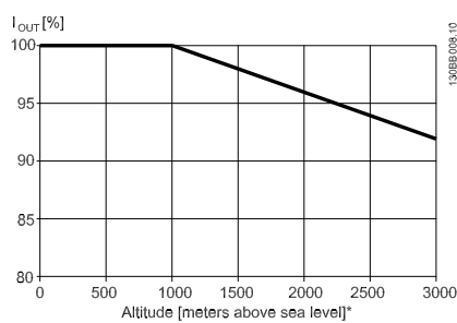
Derating da corrente de saída versus altitude na T_{AMB, MAX} para chassis de tamanhos D, E e F.
