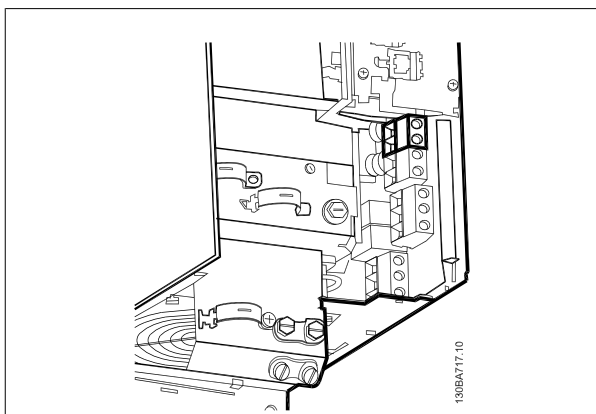
Ilustração 5.25: Conexões do barramento CC para o gabinete metálico B3..
