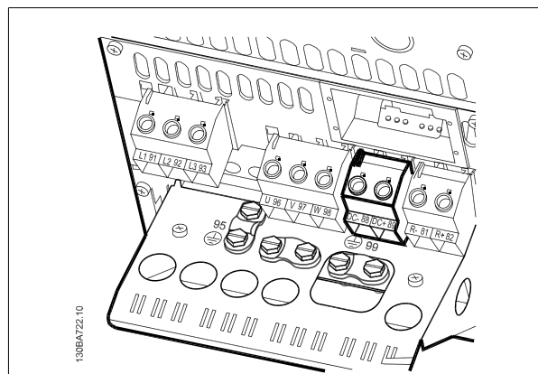
Ilustração 5.26: Conexões do barramento CC para o gabinete metálico B4.
