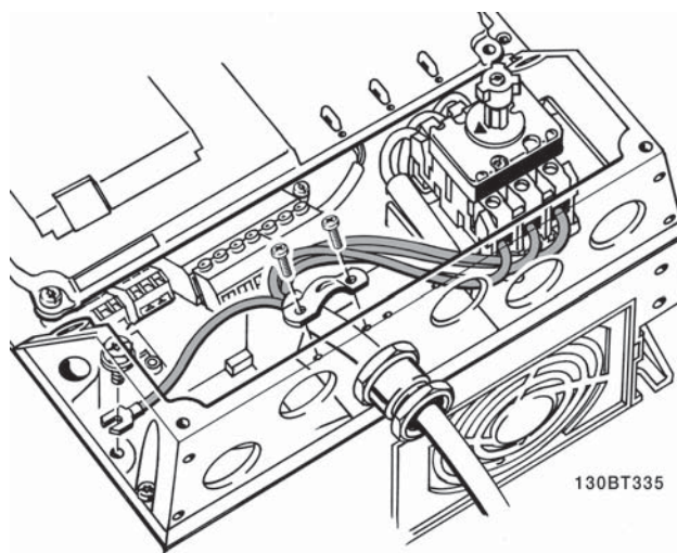
Ilustração 5.7: Como fazer a conexão à rede elétrica e ao ponto de aterramento com chave de desconexão.
