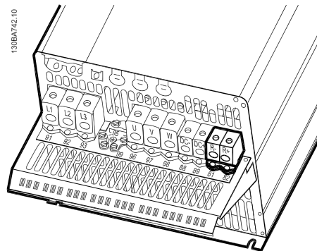
Ilustração 5.32: Terminal de conexão do freio para o C4.
