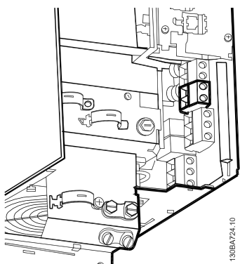
Ilustração 5.29: Terminal de conexão do freio para o B3.
