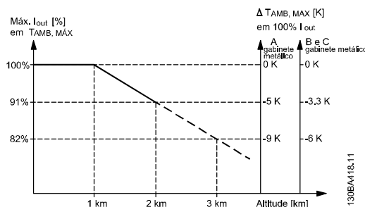
Ilustração 10.1: Derating da corrente de saída versus altitude na T_{AMB, MAX} para chassis de tamanhos A, B and C. Para altitudes acima de 2 km, entre em contacto com a Danfoss em relação à PELV.
