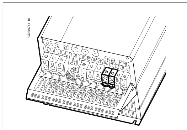
Ilustração 5.28: Conexões do barramento CC para o gabinete metálico C4
