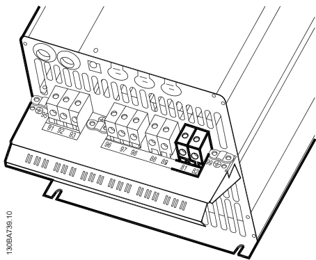
Ilustração 5.31: Terminal de conexão do freio para o C3.
