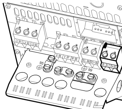
Ilustração 5.30: Terminal de conexão do freio para o B4.
