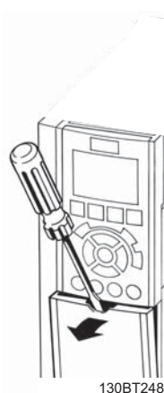
Ilustração 5.37: Acesso aos terminais de controle dos gabinetes metálicos A2, A3, B3, B4, C3 e C4
