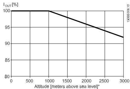
Snížení výstupního proudu v závislosti na nadmořské výšce při T_{AMB, MAX} pro velikosti rámečků D, E a F.
