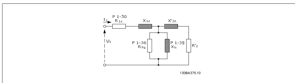
Illustration 2.1: 异步电动机的电动机当量图
