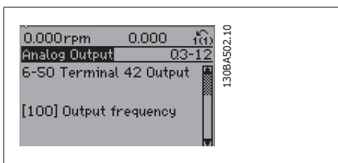
Illustration 1.7: 步骤 6: 选择参数 6-50 端子 42 输出。请按 [OK] (确定)。
