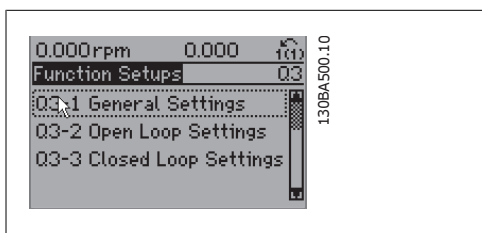
Obrázek 1.5: Krok 4: Zobrazí se možnosti menu Nastavení funkcí. Zvolte položku 03-1 Obecná nastavení . Stiskněte tlačítko [OK].
