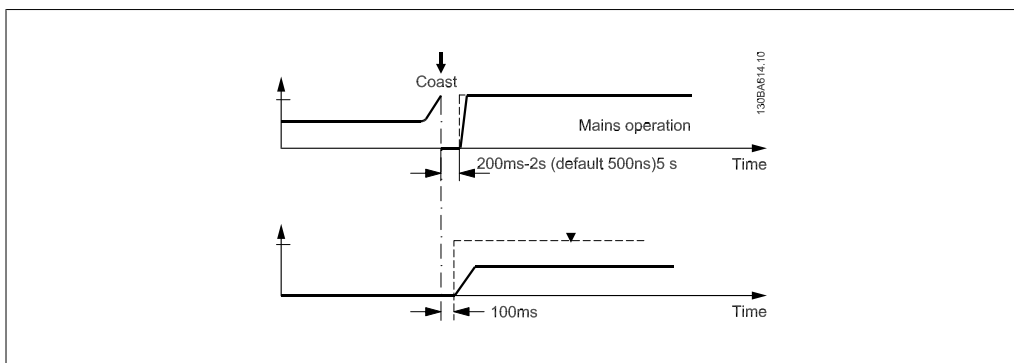
Obrázek 2.3: Konfigurace s rychlým střídáním
