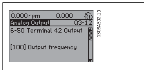
Obrázek 1.7: Krok 6: Zvolte parametr 6-50 Svorka 42, výstup . Stiskněte tlačítko [OK].
