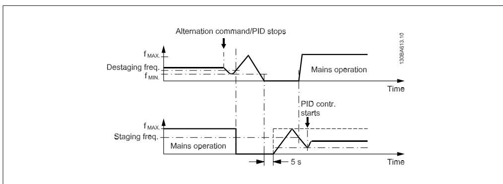
Obrázek 2.2: Konfigurace s pomalým střídáním
