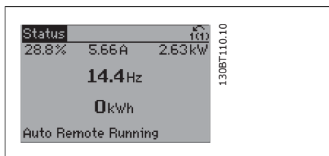
Obrázek 1.2: Krok 1: Zapněte měnič kmitočtu (rozsvítí se kontrolka On).
