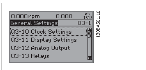
Obrázek 1.6: Krok 5: Pomocí navigačních tlačítek nahoru a dolů přejděte dolů např. na možnost 03-12 Analogové výstupy . Stiskněte tlačítko [OK].
