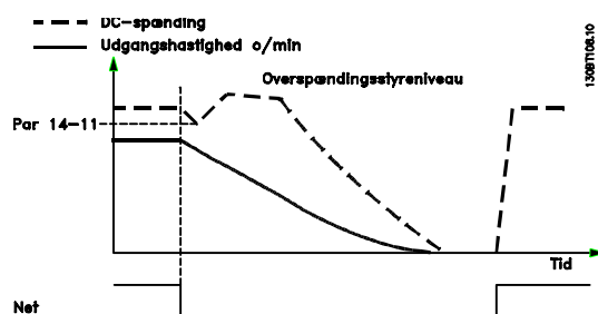
Illustration 2.3: Kontrolleret nedrampning, længere netfejl. Nedrampning så langt som energien i systemet gør det muligt, hvorefter motoren køres i friløb.
