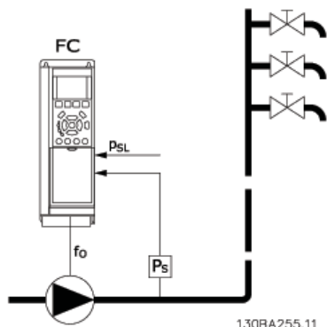
Illustration 2.6: Forklaring: FC=frekvensomformer; f_0 =frekvensudgang; P_S =P system; P_{SL} =P sætpunkt
