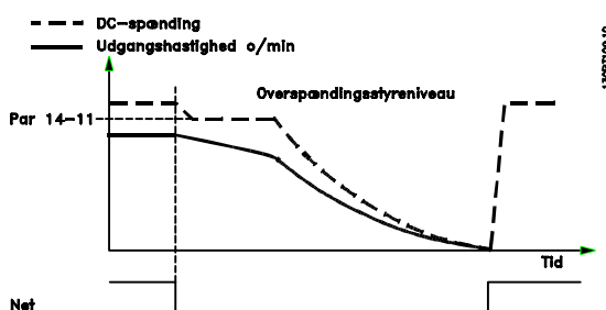
Illustration 2.5: Kinetisk backup, længere netfejl. Motoren køres i friløb, så snart energien i systemet er for lav.
