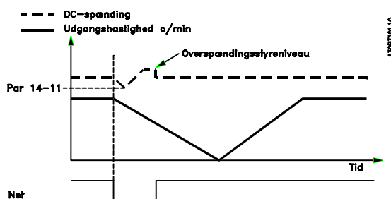
Illustration 2.2: Kontrolleret nedrampning - kort netfejl. Nedrampning til standsning efterfulgt af en oprampning til referencen.
