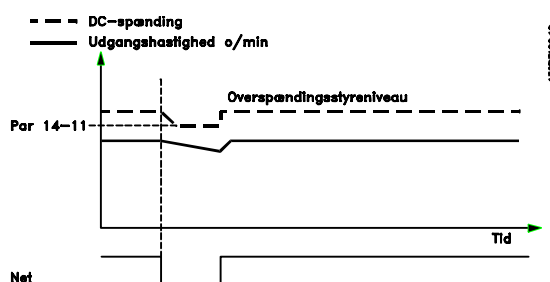
Illustration 2.4: Kinetisk backup, kort netfejl. Kør igennem så længe energien i systemet gør det muligt.
