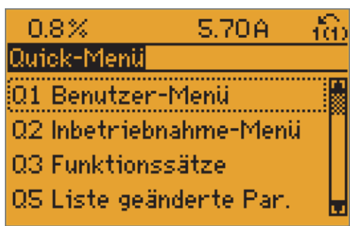
Abbildung 5.1: Quick-Menü-Anzeige
