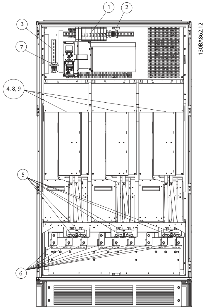
Abbildung 3.47: Wechselrichtergehäuse, Baugröße F2 und F4
