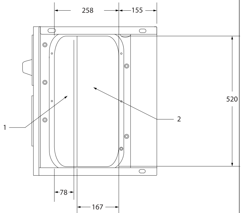
Ansicht der Kabeleinführungen von der Unterseite des Frequenzumrichters – 1) Netzseite 2) Motorseite
