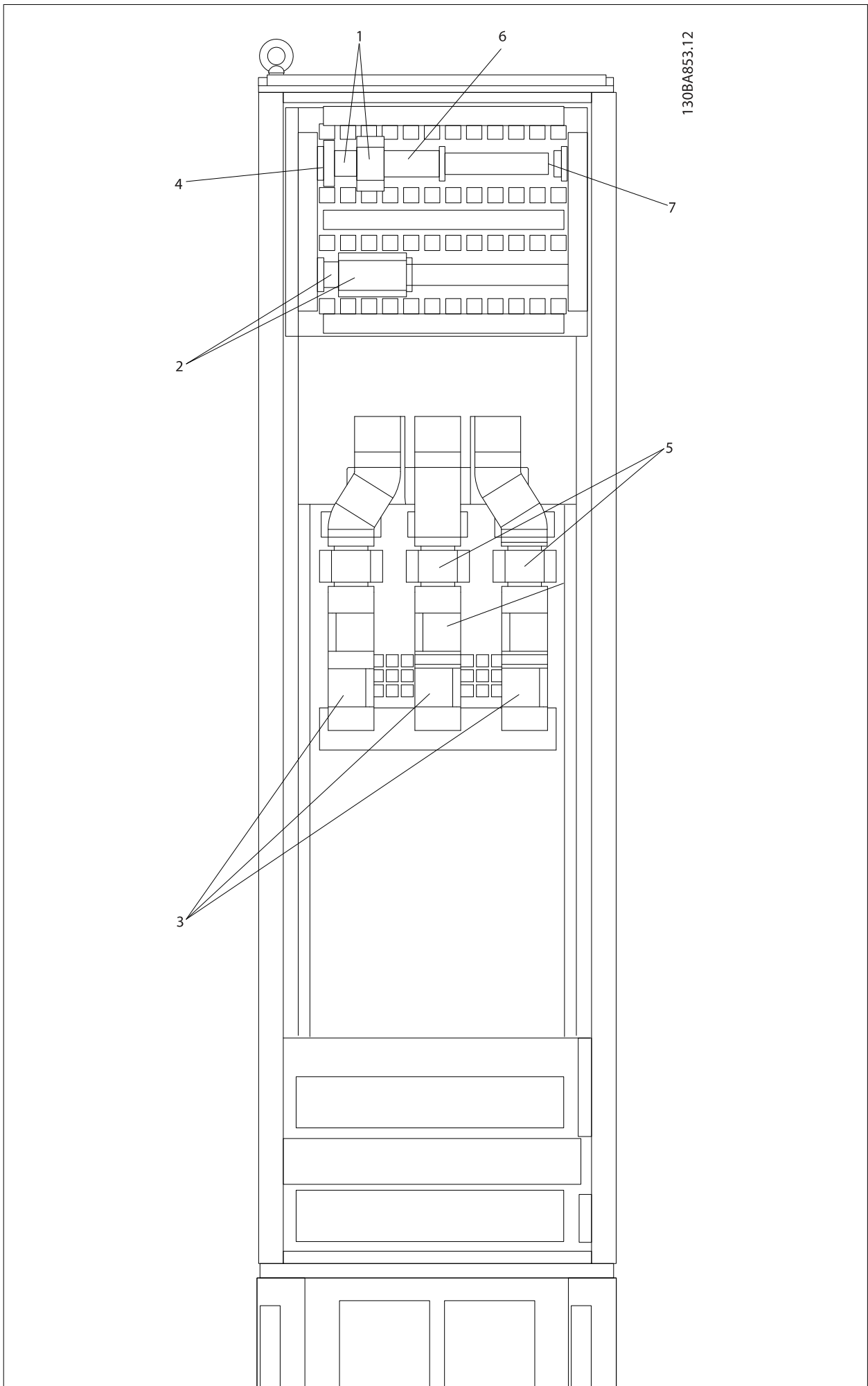
Abbildung 3.48: Optionsgehäuse, Baugröße F3 und F4
