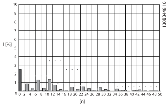
Ilustración 3.2: Espectro de frecuencia de armónicos habitual y valor THD en los terminales de red del convertidor de frecuencia n = orden de armónicos límites ◇.....IEEE519 ( I_{sc} / I_L > 20 ) para armónicos individuales
