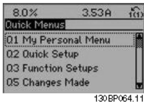
Afbeelding 6.1: Overzicht snelmenu
