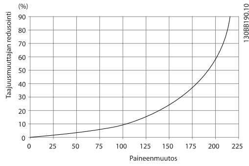
Kuva 4.23: F-kehksen redusointi vrt. paineenmuutos Taajuusmuuttajan ilmavirtaus: 580 cfm (985 m 3 /h)
