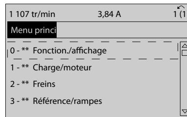
Illustration 6.9 Exemple d'affichage.
