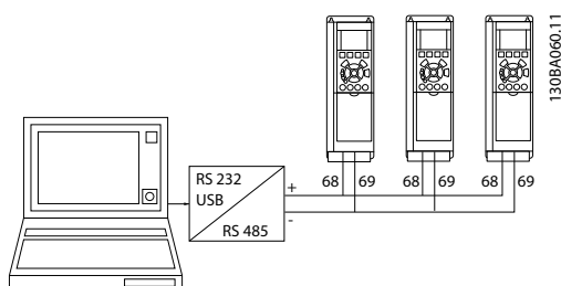
Kuva 5.9 Kytchentäesimerkki.
