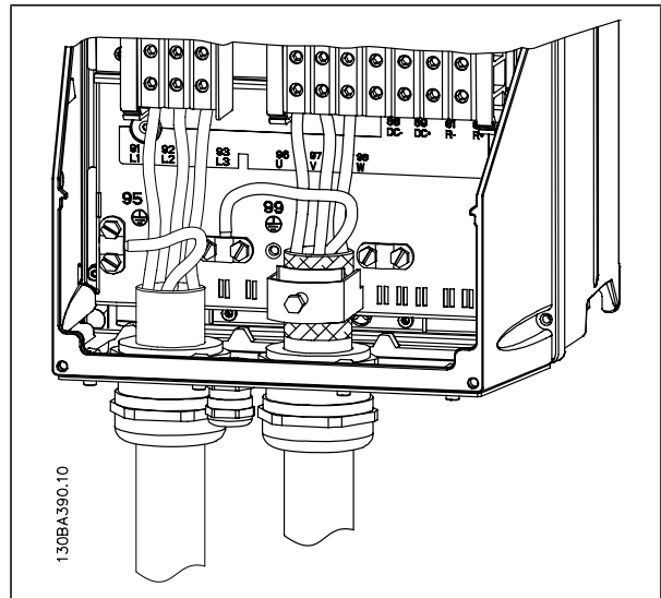
C1 和 C2 (IP 21/NEMA 类型 1 和 IP 55/66/NEMA 类型 12) 机箱的电动机连接
