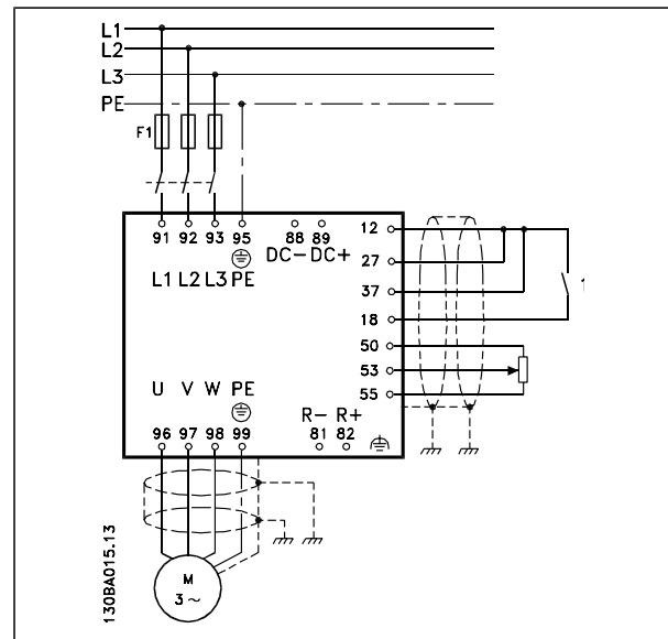
此图显示了基本安装，其中包括主电源、电动机、启动/停止键以及用于调整转速的电位计。
