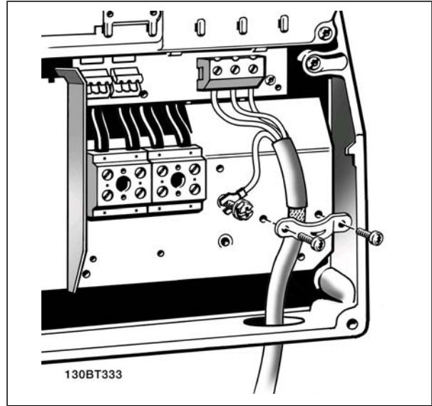
B1 和 B2 (IP 21/NEMA 类型 1、IP 55/ NEMA 类型 12 和 IP66/ NEMA 类型 4X) 机箱的电动机连接
