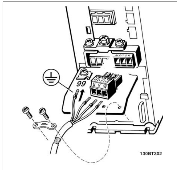
A1、A2 和 A3 的电动机连接
