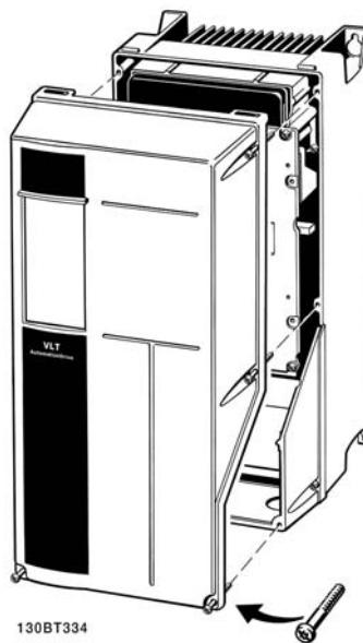
図 3.20: A5、B1、B2、C1、C2 エンクロージャのコントロール端子にアクセス
