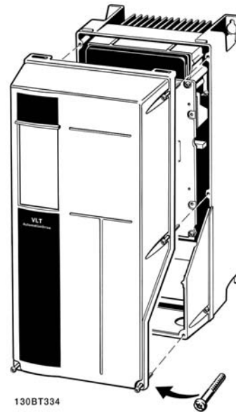
그림 3.19: A5, B1,B2, C1 및 C2 외함의 제어 단자 접근 방법
