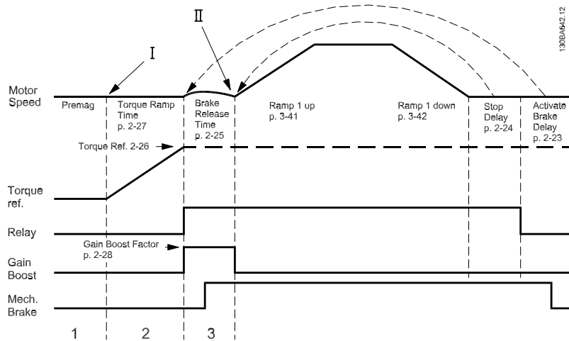
그림 4.1: 호이스트 기계식 제동장치 제어를 위한 제동 해제 시퀀스
