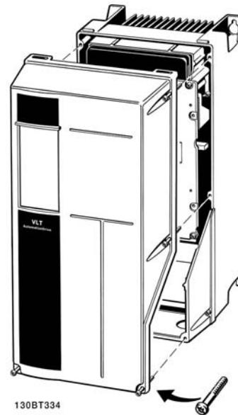
図 3.19: A5、B1、B2、C1、C2 エンクロージャのコントロール端子にアクセス
