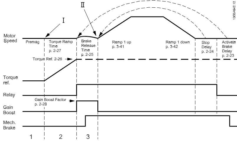
図 4.1: 巻き上げ機械的ブレーキ・コントロールのブレーキ解放手順
