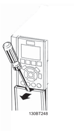
圖 3.18: 操作 A2、A3、B3、B4、C3 與 C4 外殼的控制端子
