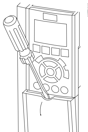
Obrázek 3.20: Přístup k řídicím svorkám pro krytí A2, A3, B3, B4, C3 a C4
