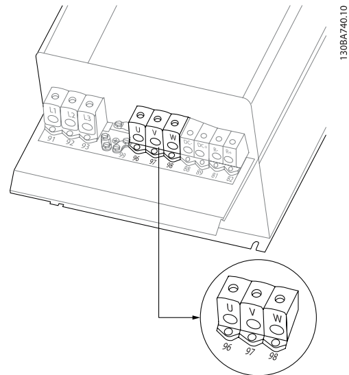
Obrázek 3.15: Připojení k motoru pro velikosti rámečků C3 a C4.
