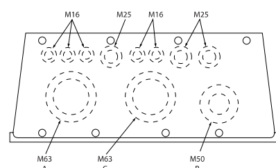
Obrázek 3.19: Otvory pro kabely pro velikost rámečku C2. Navrhované umístění otvorů je pouze doporučení a je možné použít i jiná řešení.
