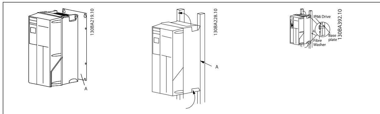
Tabulka 3.1: Při montáži rámečků velikosti A4, A5, B1, B2, C1 a C2 na nepevnou stěnu musí být měnič vybaven zadní deskou A kvůli nedostatečnému průchodu chladicího vzduchu nad chladičem.
