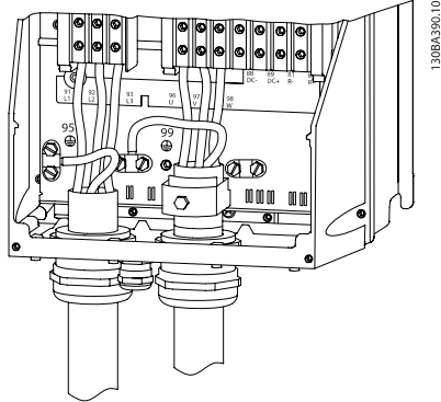
Obrázek 3.14: Připojení k motoru pro velikosti rámečků C1 a C2 (IP 21/ NEMA typ 1 a IP 55/66/ NEMA typ 12)
