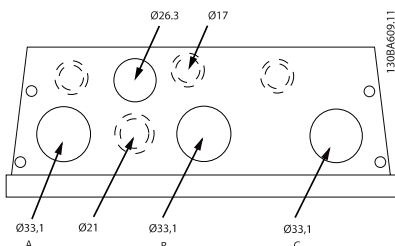
Obrázek 3.16: Otvory pro kabely pro velikost rámečku B1. Navrhované umístění otvorů je pouze doporučení a je možné použít i jiná řešení.
