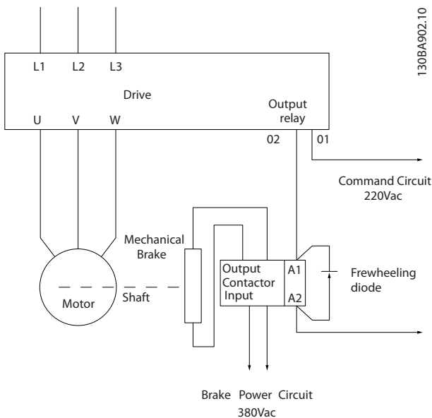
圖 2.17 將機械煞車連接至變頻器
