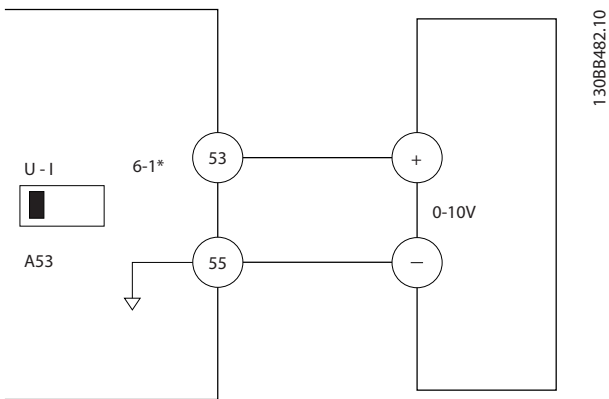
圖 5.1 提供 0-10V 控制信號之外部裝置的配線範例 (左為變頻器，右為外部裝置)
