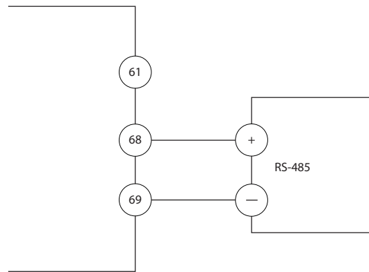
圖 2.18 串列通訊配線圖
