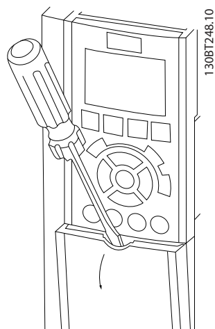
Ilustracja 2.9 Dostęp do okablowania sterowania dla obudów A2, A3, B3, B4, C3 i C4.
