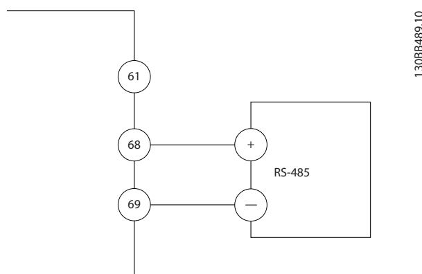
Ilustracja 2.18 Schemat połączeń elektrycznych komunikacji szeregowej
