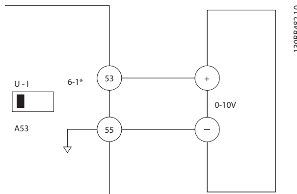
Ilustracja 5.1 Przykład połączeń elektrycznych dla urządzenia zewnętrznego dostarczającego sygnał sterujący 0-10 V (przetwornica częstotliwości po lewej, urządzenie zewnętrzne po prawej)
