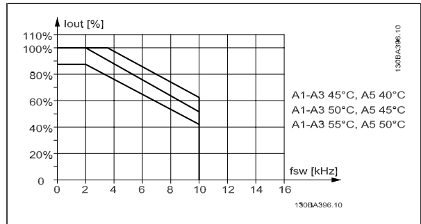
I_{out} 在不同 T_{AMB, MAX} 下的降容 - A 型机箱，开关模式为 SFAVM，电动机电缆的最大长度不超过 10 m
