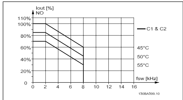
I_{out} 在不同 T_{AMB, MAX} 下的降容 - C 型机箱, 在正常转矩模式 (110% 过转矩) 下使用 SFAVM
