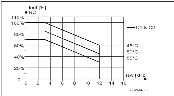
I_{out} 在不同 T_{AMB, MAX} 下的降容 - C 型机箱, 在正常转矩模式 (110% 过转矩) 下使用 60 PWM
