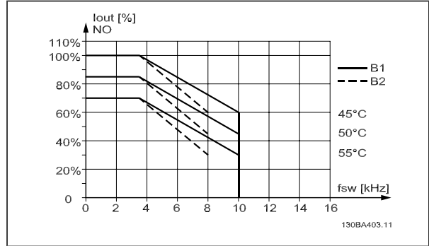
I_{out} 在不同 T_{AMB, MAX} 下的降容 - B 型机箱, 在正常转矩模式 (110% 过转矩) 下使用 SFAVM
