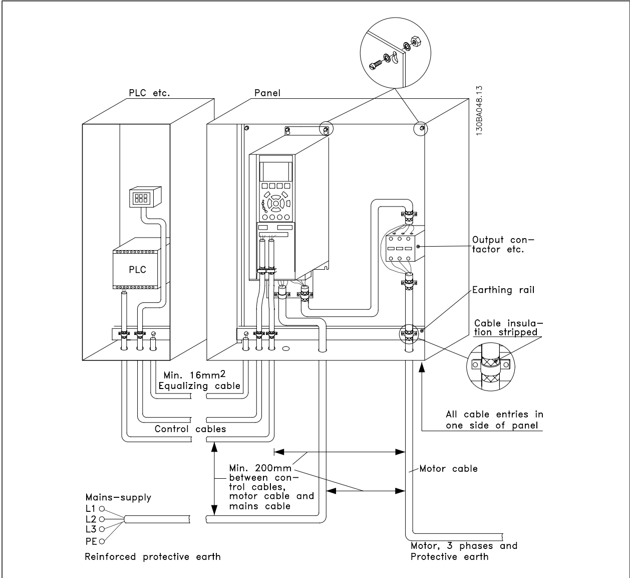
IP20 变频器符合 EMC 规范的电气安装。
