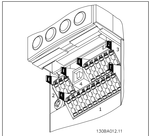
控制端子（所有机箱）
