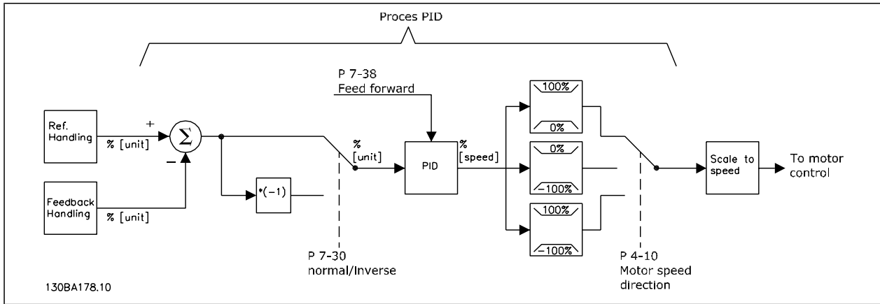
过程 PID 控制图
