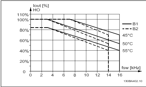
I_{out} 在不同 T_{AMB, MAX} 下的降容 - B 型机箱, 在高转矩模式 (160% 过转矩) 下使用 60 PWM
