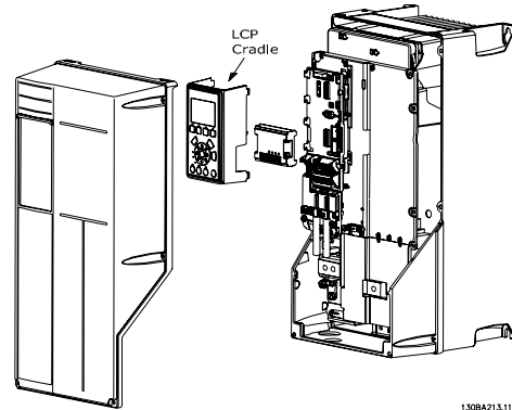
A5、B1、B2、C1 和 C2 规格的机架
