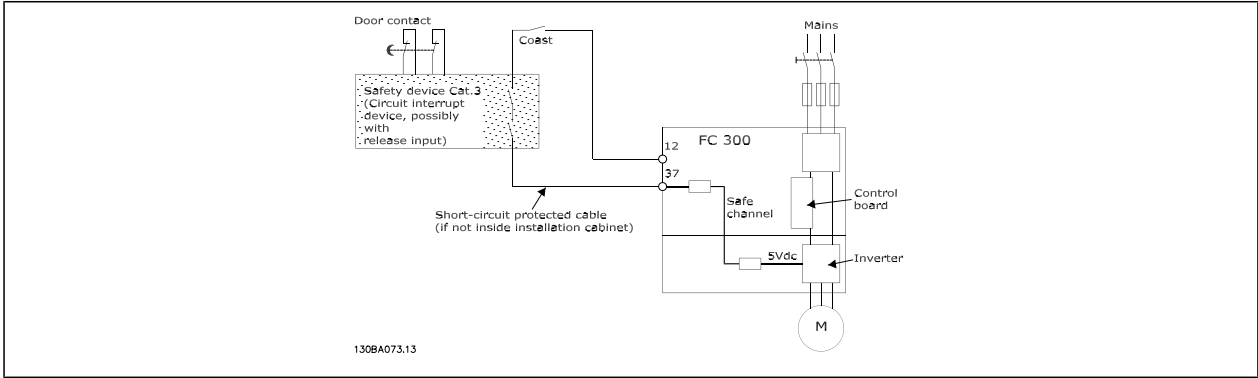
符合安全类别 3 (EN 954-1) 停止类别 0 (EN 60204-1) 的安装基本配置的简图。
