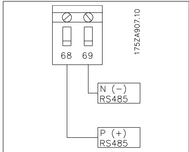
网络端子连接
