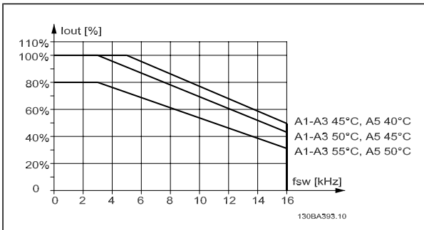
I_{out} 在不同 T_{AMB, MAX} 下的降容 - A 型机箱，开关模式为 60 PWM
