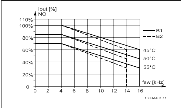
I_{out} 在不同 T_{AMB, MAX} 下的降容 - B 型机箱, 在正常转矩模式 (110% 过转矩) 下使用 60 PWM
