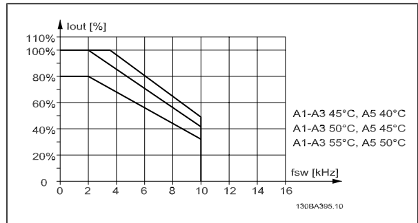
I_{out} 在不同 T_{AMB, MAX} 下的降容 - A 型机箱，开关模式为 SFAVM
