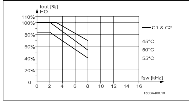
I out 在不同 T AMB, MAX 下的降容 - C 型机箱, 在高转矩模式 (160% 过转矩) 下使用 SFAVM
