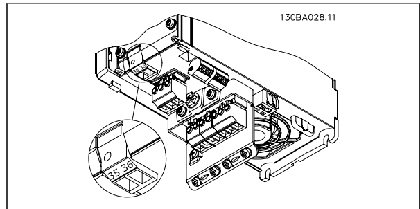
A2 和 A3 规格机架上 24 V 备用电源的连接。
