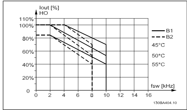
I_{out} 在不同 T_{AMB, MAX} 下的降容 - B 型机箱, 在高转矩模式 (160% 过转矩) 下使用 SFAVM
