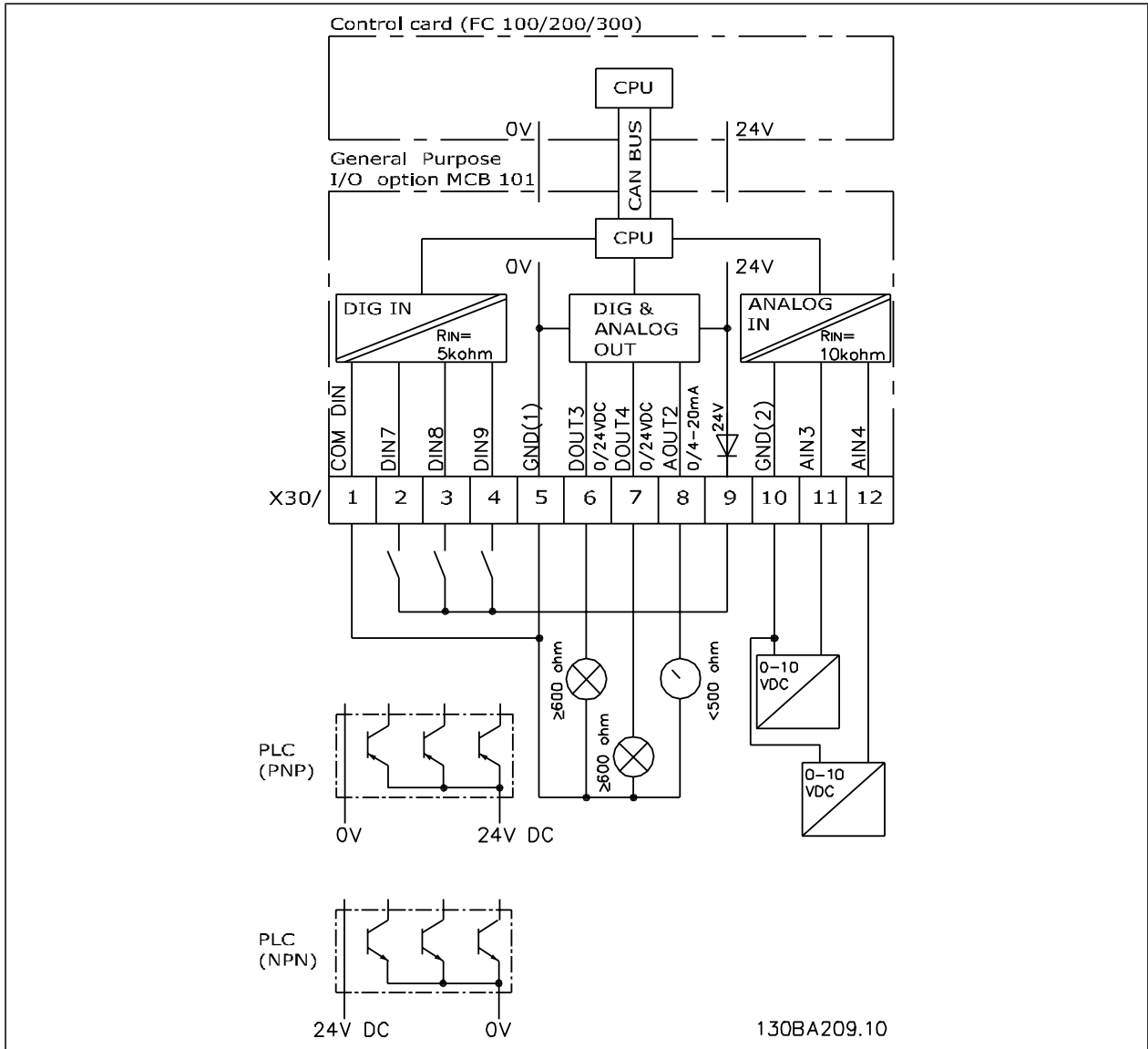
原理图
