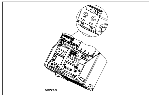
A5、B1、B2、C1 和 C2 规格机架上 24 V 备用电源的连接。
