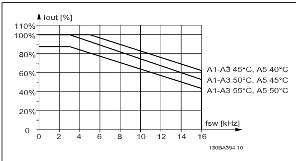
I_{out} 在不同 T_{AMB, MAX} 下的降容 - A 型机箱，开关模式为 60 PWM，电动机电缆的最大长度不超过 10 m
