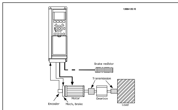
FC 302 闭环速度控制的基本设置
