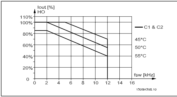
I out 在不同 T AMB, MAX 下的降容 - C 型机箱, 在高转矩模式 (160% 过转矩) 下使用 60 PWM
