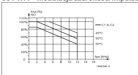
Ilustracja 4.9: Obniżanie wartości znamionowych I_{out} dla różnych T_{AMB, MAX} dla obudowy C za pomocą 60 PWM w trybie wysokiego momentu obrotowego (obrót maks. 160%)
