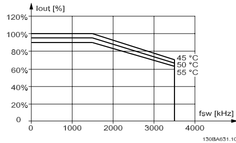
图 4.22: 690 V 时, I_{out} 在不同 T_{AMB, MAX} 下的降容 - D 型机箱, 在高转矩模式 (160% 过转矩) 下使用 SFAVM。注意: 仅限 P315。
