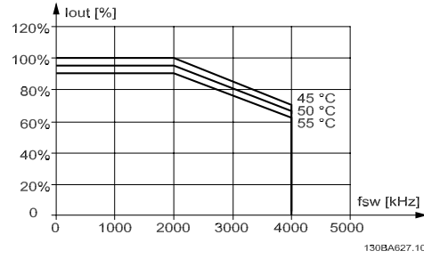
图 4.18: 690 V 时, I_{out} 在不同 T_{AMB, MAX} 下的降容 - D 型机箱, 在高转矩模式 (160% 过转矩) 下使用 SFAVM。注意: 对 P315 无效。
