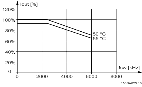
图 4.17: 690 V 时, I_{out} 在不同 T_{AMB, MAX} 下的降容 - D 型机箱, 在高转矩模式 (160% 过转矩) 下使用 60 PWM。注意: 对 P315 无效。
