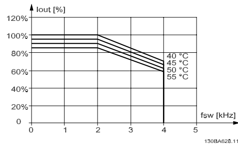
图 4.20: 690 V 时, I_{out} 在不同 T_{AMB, MAX} 下的降容 - D 型机箱, 在正常转矩模式 (110% 过转矩) 下使用 SFAVM。注意: 对 P315 无效。
