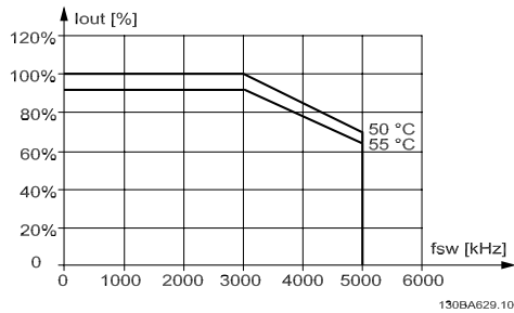
图 4.21: 690 V 时, I_{out} 在不同 T_{AMB, MAX} 下的降容 - D 型机箱, 在高转矩模式 (160% 过转矩) 下使用 60 PWM。注意: 仅限 P315。
