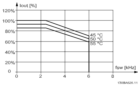
图 4.19: 690 V 时, I_{out} 在不同 T_{AMB, MAX} 下的降容 - D 型机箱, 在正常转矩模式 (110% 过转矩) 下使用 60 PWM。注意: 对 P315 无效。
