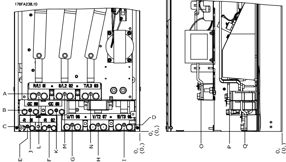
图 6.4: 电源连接的位置, D3/D4 机箱
