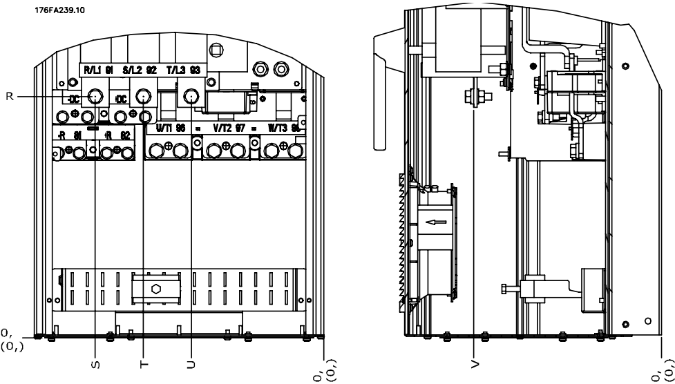
图 6.5: 断路器的电源接头位置, D1/ D2 机箱
