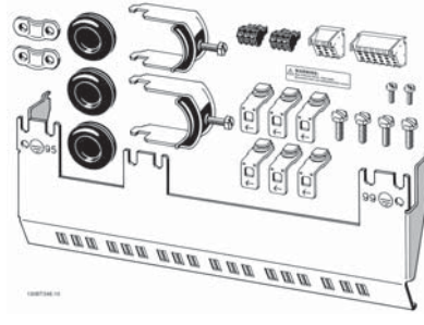
Типоразмер корпуса В3, IP20/Шасси
