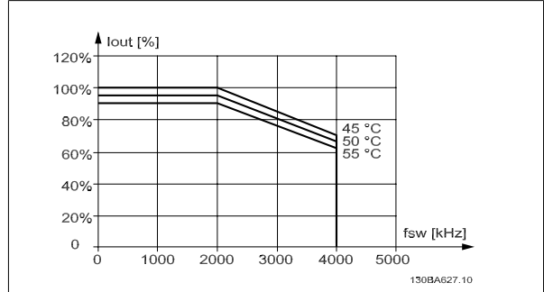
Рисунок 4.18: Снижение тока I_{out} для различных значений T_{AMB, MAX} для корпуса D при напряжении 690 В при использовании модели коммутации SFAVM в режиме высокого крутящего момента (перегрузка по крутящему моменту 160 %). Примечание: не действительно для P315.
