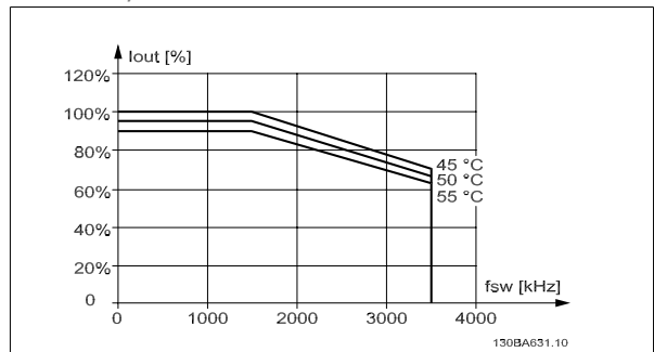
Рисунок 4.22: Снижение тока I_{out} для различных значений T_{AMB, MAX} для корпуса D при напряжении 690 В при использовании модели коммутации SFAVM в режиме высокого крутящего момента (перегрузка по крутящему моменту 160 %). Примечание: только для P315.
