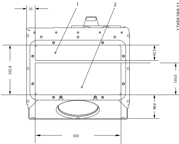
Illustration 7.45 Frame Sizes D1 + D2
