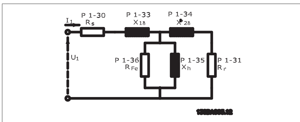
Illustration 2.1: Diagramme d'équivalence moteur pour un moteur asynchrone
