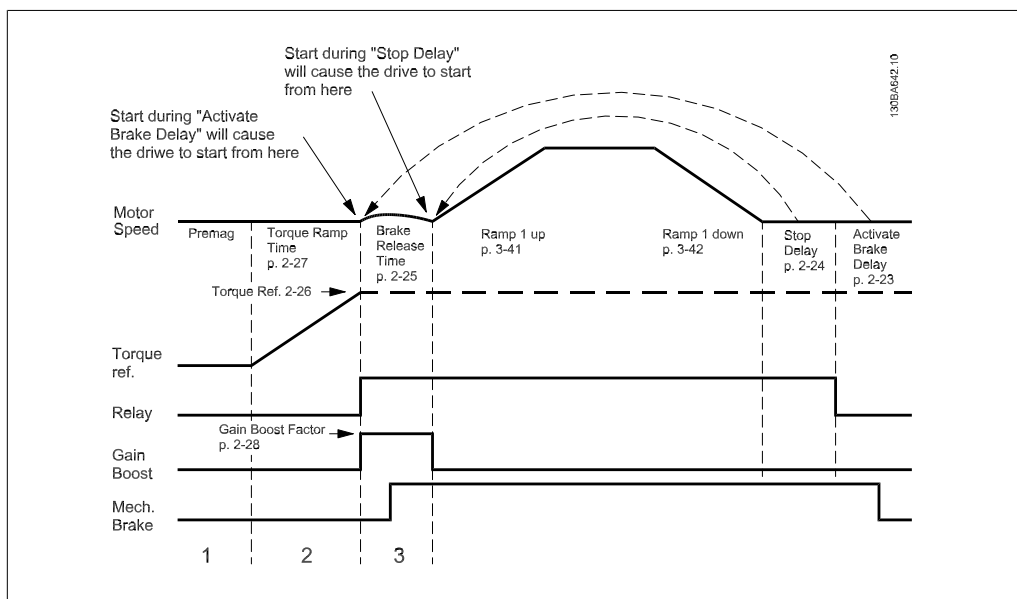
Illustration 2.4: Séquence de déclenchement du frein pour la commande de frein mécanique pour levage
