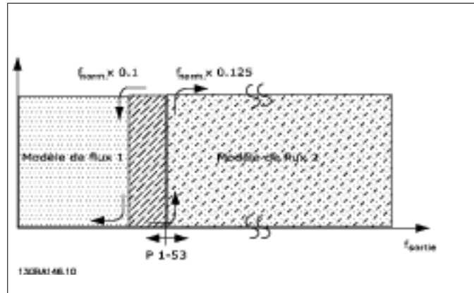
Illustration 2.2: Par. 1-00 = Boucle fermée vit. [1] ou Couple [2] et par. 1-01 = Flux retour codeur [3]
