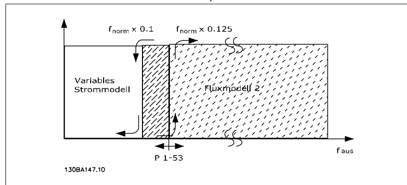
Abbildung 3.3: Par. 1-00 = [0] Drehzahl ohne Rückf., Par. 1-01 = [2] Fluxvektor oh. Geber
