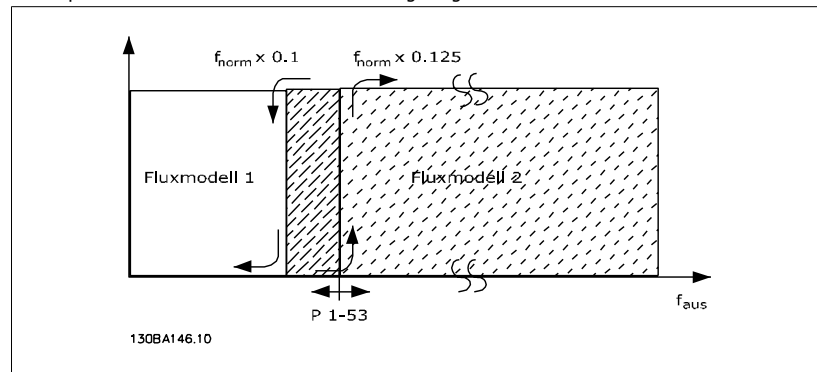
Abbildung 3.2: Funktion bei Fluxvektor mit Geber Par. 1-01 = [3]
