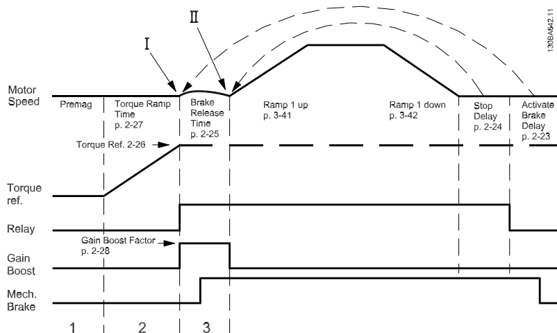
图 3.4: 起重机械制动控制的抱闸释放过程
