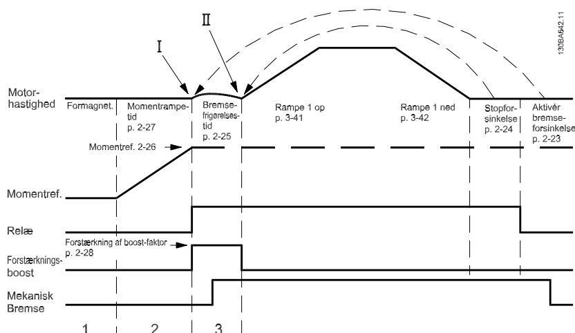
Illustration 3.6: Bremsefrigørelsessekvens for hæve/sænkemekanisk bremsestyring
