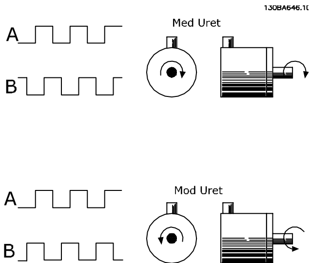
Illustration 3.5: 24 V trinvis encoder. Maks. kabellængde 5 m.
