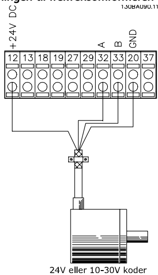
Illustration 3.5: 24 V trinvis encoder. Maks. kabellængde 5 m.
