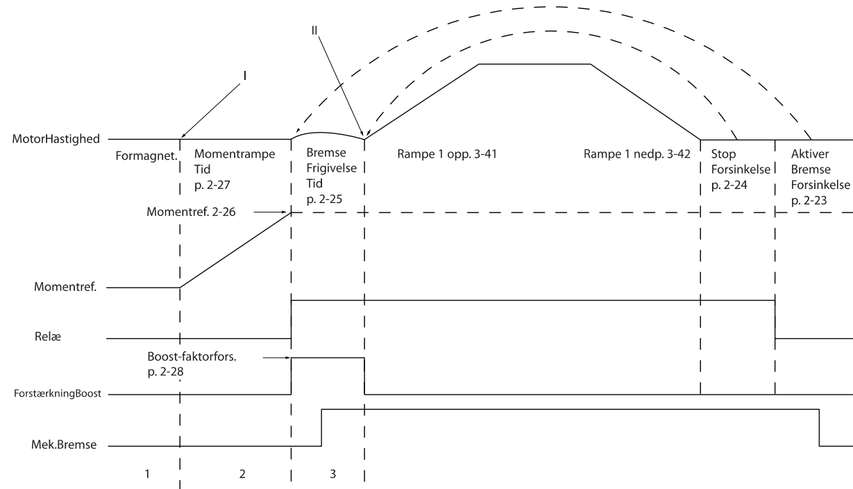
Illustration 3.4: Bremsefrigørelsessekvens for hæve/sænkemekanisk bremsestyring
