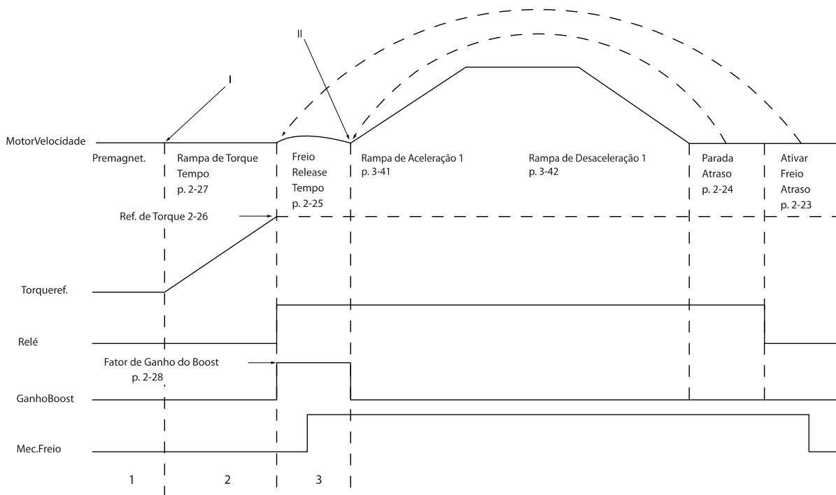
Ilustração 3.5 Sequência de liberação do freio para controle do freio mecânico do içamento
