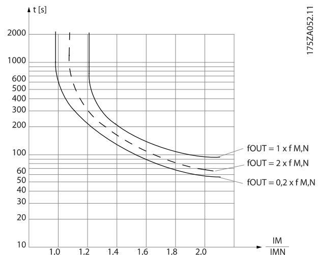
Ilustração 3.4 Perfil ETR
