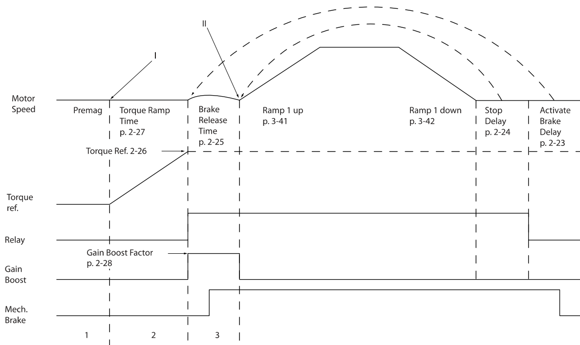
Рисунок 3.5 Последовательность отпусания тормоза при управлении механическим тормозом подъемного механизма
