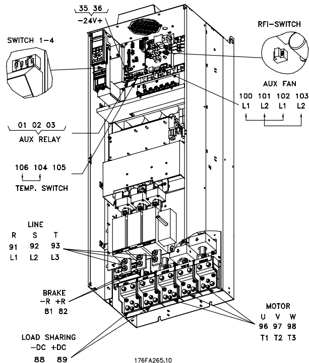
Compact IP 00 med fränskiljare och säkring VLT 5352-5552 380-500 V, VLT 5402-5602 525-690 V
