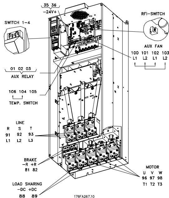
Compact IP 00 utan fränskiljare och säkring VLT 5352-5552 380-500 V, VLT 5402-5602 525-690 V Observera: RFI-switchen fungerar inte i 525-690 V-frekvensomformare.
