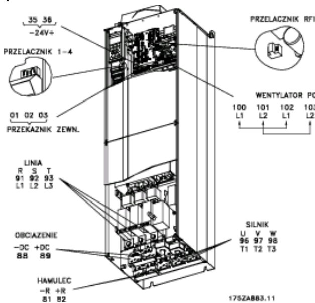
Kompakt IP 21/IP 54 z rozłącznikiem i bezpiecznikiem VLT 5202-5302 380-500 V, VLT 5202-5352 525-690 V Uwaga: Przelącznik RFI nie ma funkcji w przetwornicach 525-690 V
