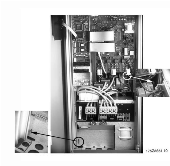
Kompakt IP 54 VLT 5008 - 5011 200 - 240 V VLT 5016 - 5027 380 - 500 V
