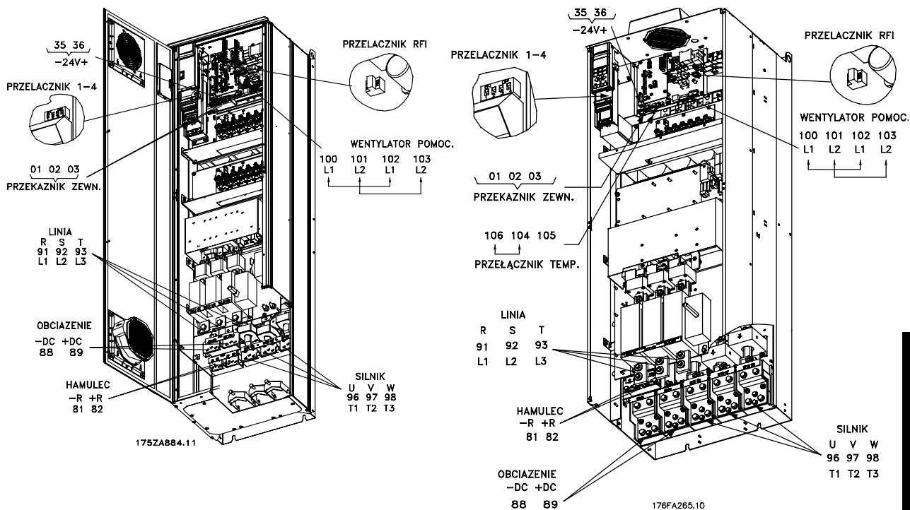
Kompakt IP 21/IP 54 z rozłącznikiem i bezpiecznikiem VLT 5202-5302 380-500 V, VLT 5202-5352 525-690 V Uwaga: Przelącznik RFI nie ma funkcji w przetwornicach 525-690 V
