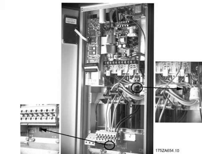
Kompakt IP 54 VLT 5016 - 5027 200 - 240 V VLT 5032 - 5062 380 - 500 V
