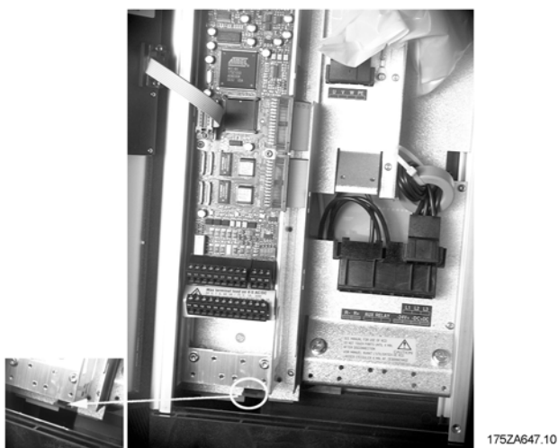
Compact IP 54 VLT 6002 - 6011 380 - 460 V VLT 6002 - 6005 200 - 240 V
