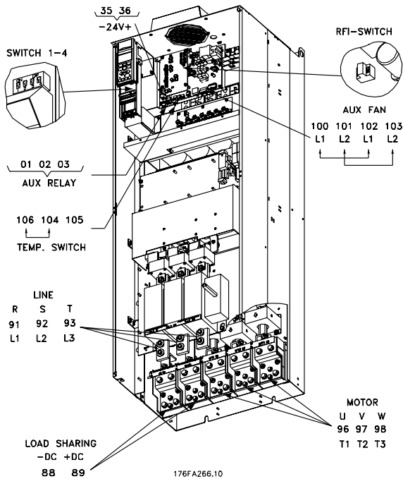
Compact IP 00 med afbryder og sikring VLT 6402-6602 380-460 V og VLT 6502-6652 525-600 V
