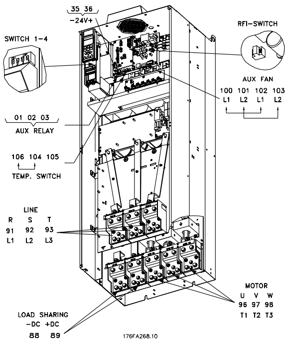
Compact IP 00 uden afbryder og sikring VLT 6402-6602 380-460 V og VLT 6502-6652 525-600 V
