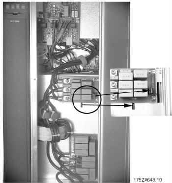
Compact IP 20/NEMA 1 VLT 8052-8122 380-480 V VLT 8027-8032 200-240 V VLT 8052-8072 525-600 V
