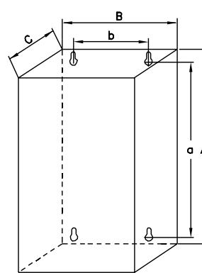
Typ G, IP54
