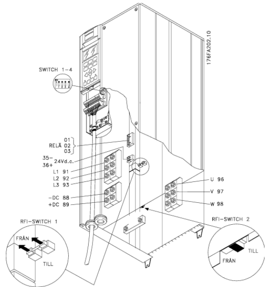
Compact IP 00/Chassi VLT 8042-8062, 200-240 V
