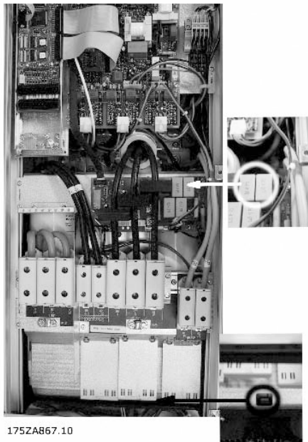
Compact IP 54/NEMA 12 VLT 8102-8122 380-480 V
