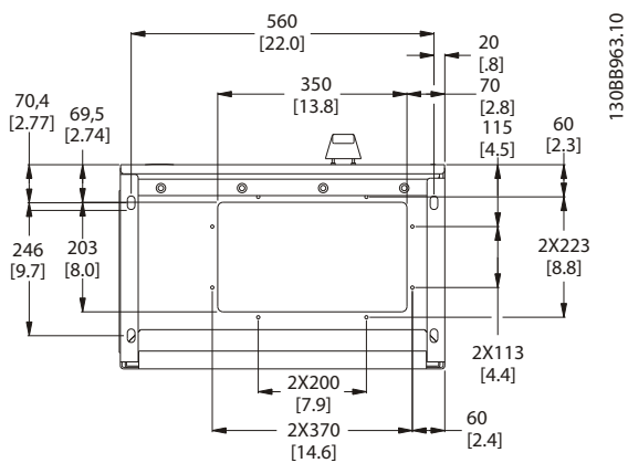
Ilustración 4.19 Tamaño del bastidor D13
