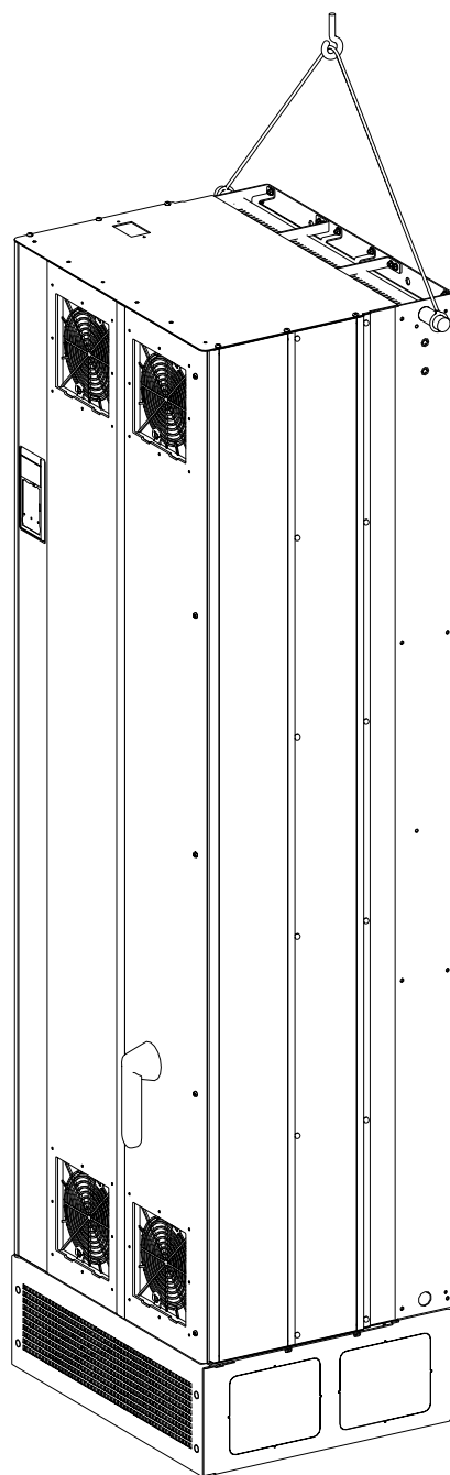
Ilustración 4.3 Método de elevación recomendado para AAF 006, tamaños del bastidor D13 y E9.
