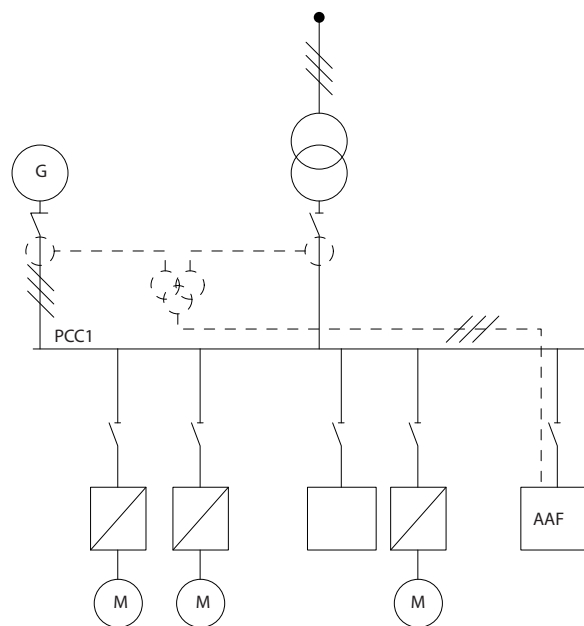
Ilustración 4.34 CT sumadores en aplicaciones de respaldo de generadores (lado de PCC). El filtro compensa la corriente completa de transformador y generador.
