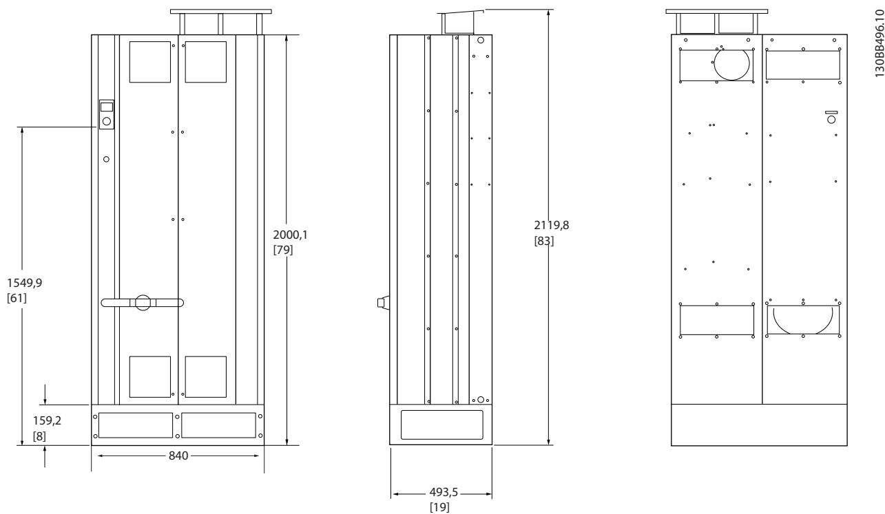
Ilustración 4.6 Tamaño del bastidor E7, AAF05
