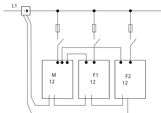
Ilustración 4.44 Diagrama de conexión de CT de una fase para maestro y auxiliar.
