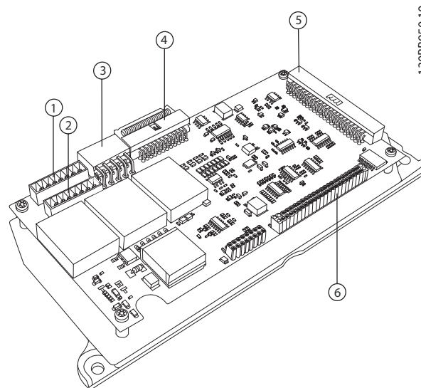
Ilustración 4.29 Placa AFC
