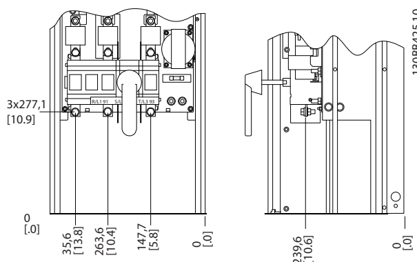
Ilustración 4.12 Ubicación del terminal del bastidor D9
