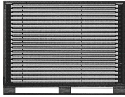
B-B 1:14
